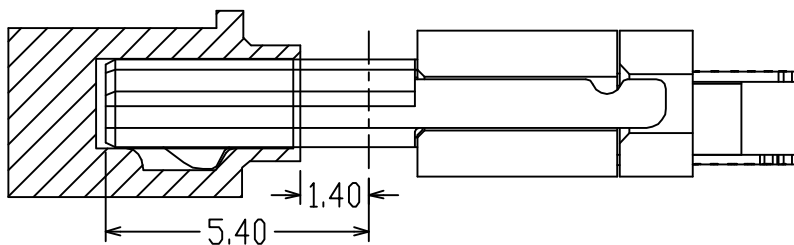
B-B剖视图
